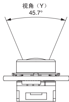
视角（Y方向）
