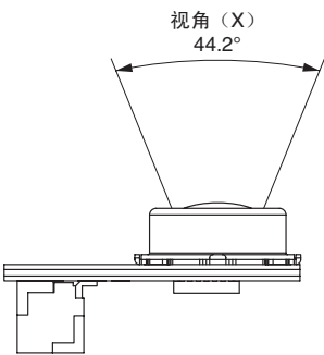
视角（X方向）
