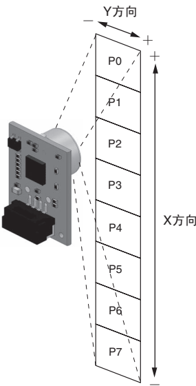
各像素的检测区域
