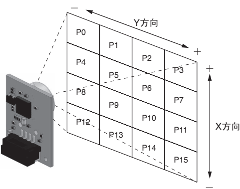
各像素的检测区域
