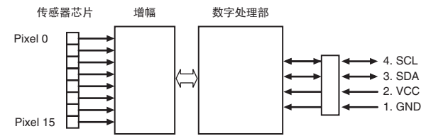
温度传感器结构图
